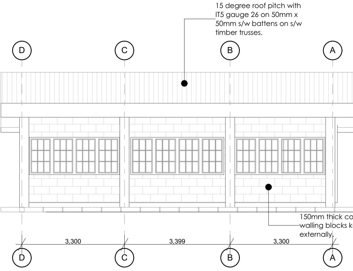
ELEVATION E-04 1:75
