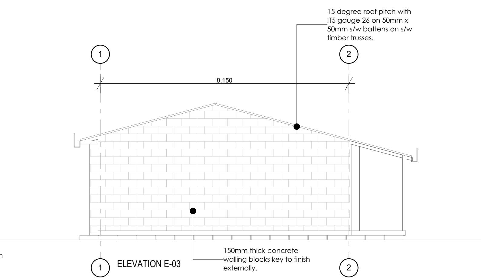
ELEVATION E-03 1:75
