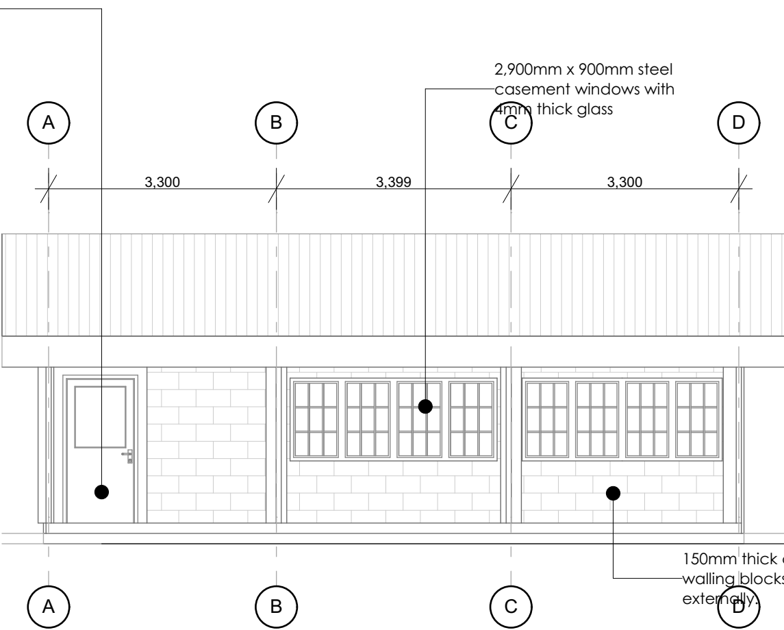
ELEVATION E-02 1:75
