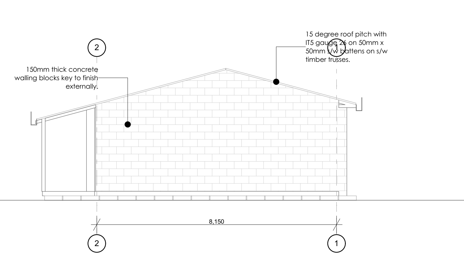
ELEVATION E-05 1:75
