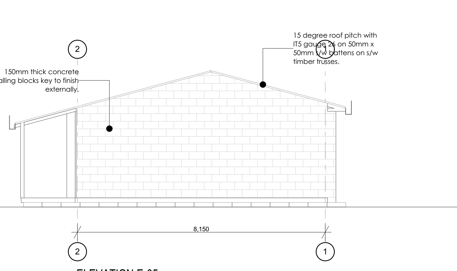
ELEVATION E-05 1:75
