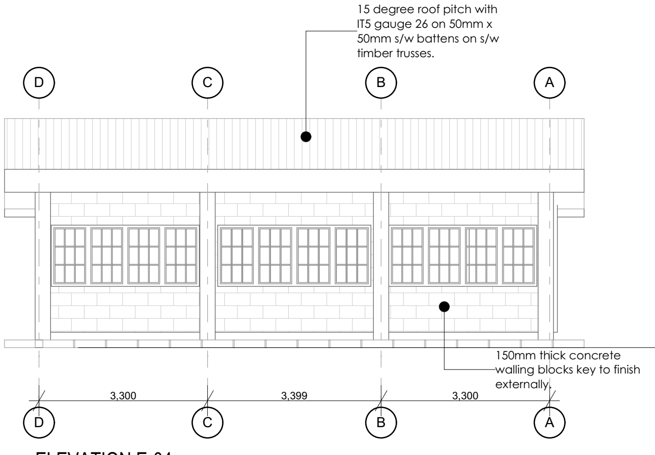
ELEVATION E-04 1:75
