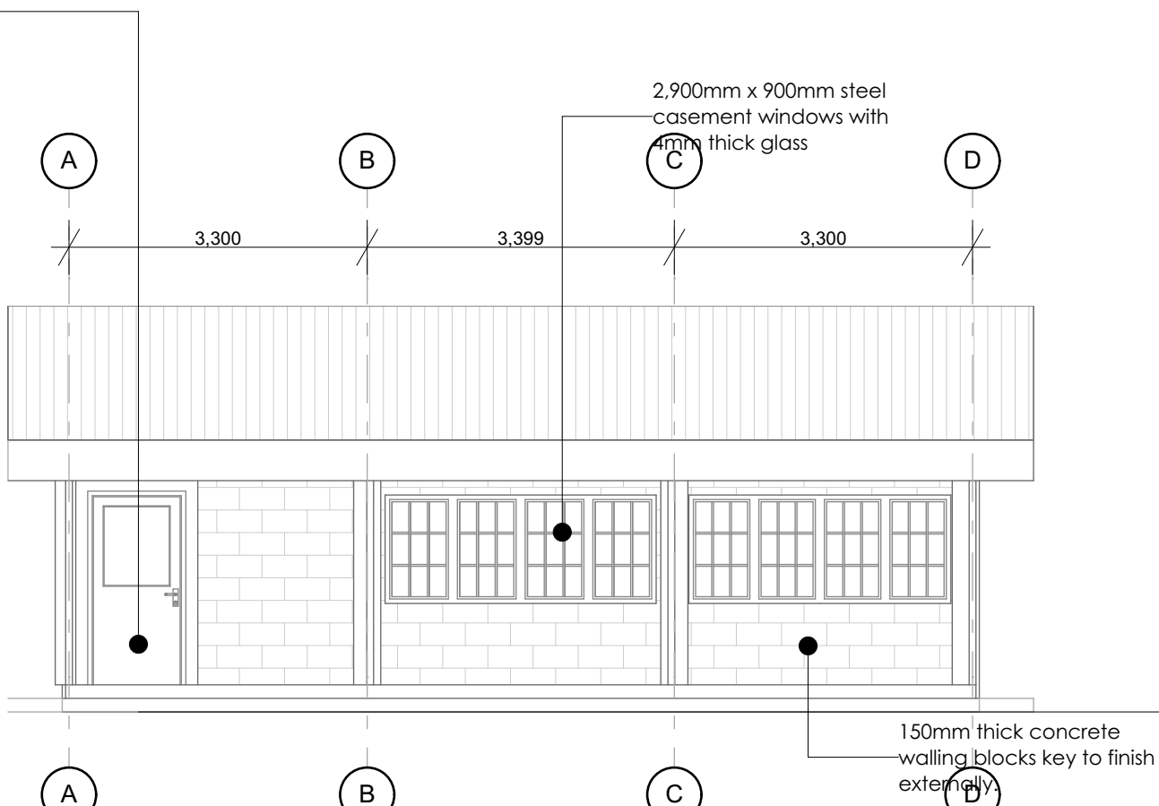
ELEVATION E-02 1:75
