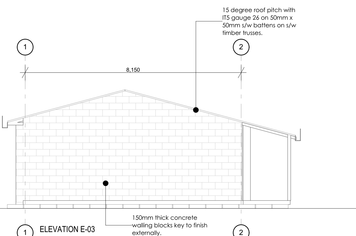
ELEVATION E-03 1:75
