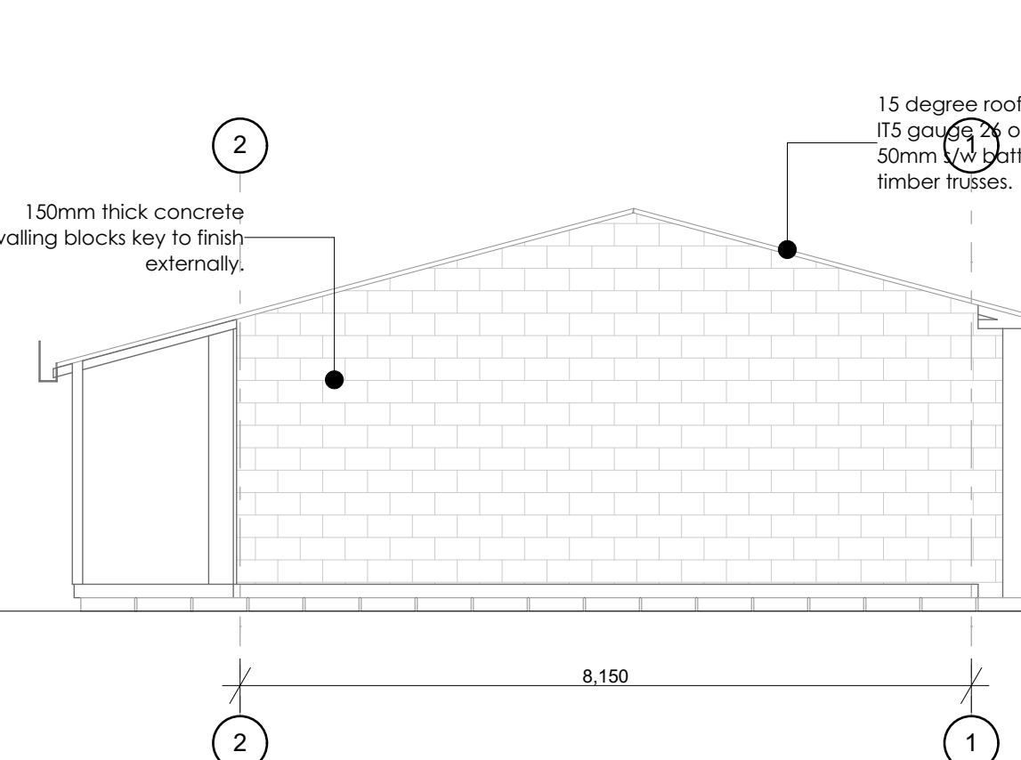
ELEVATION E-05 1:75
