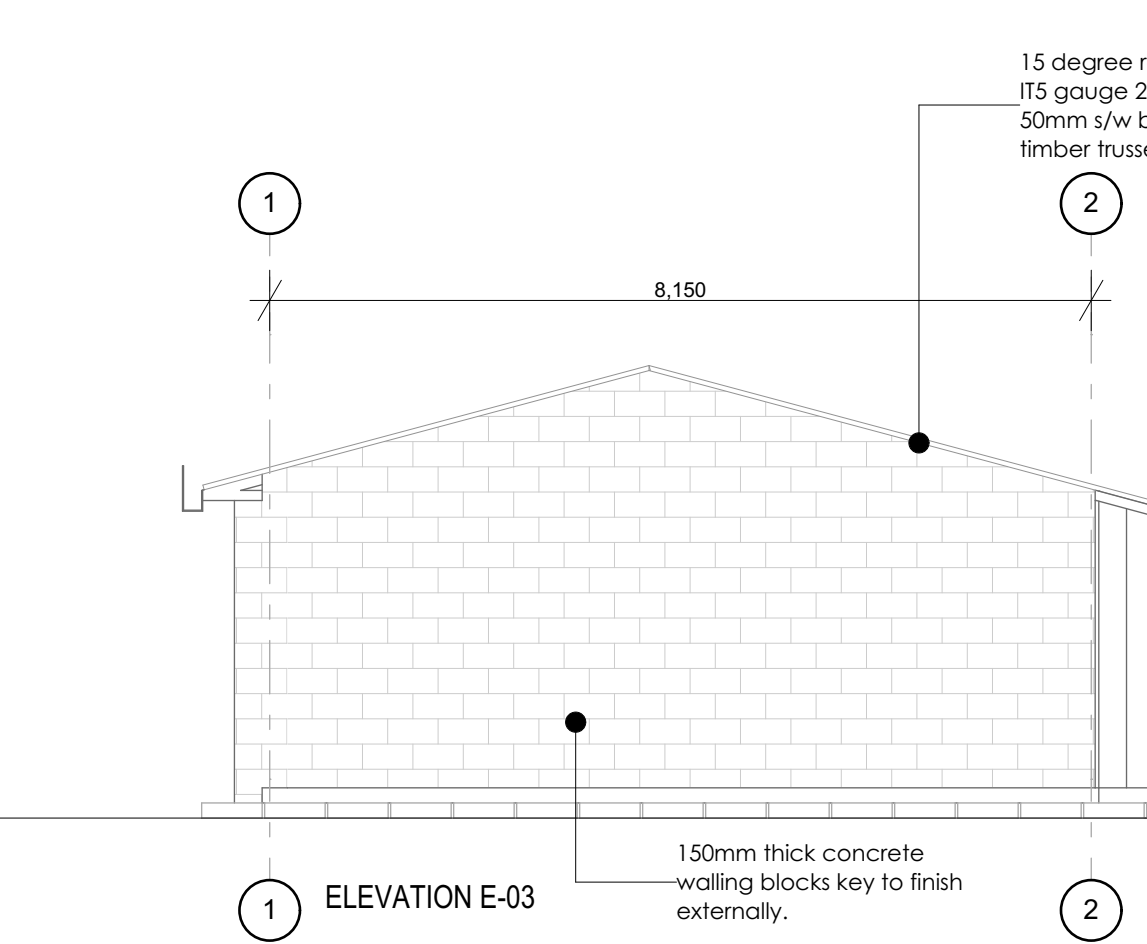
ELEVATION E-03 1:75
