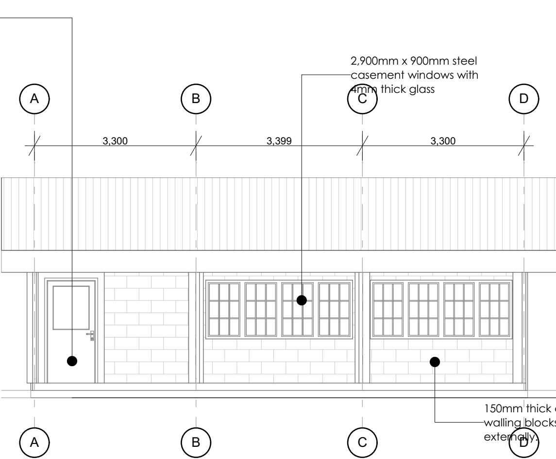
ELEVATION E-02 1:75
