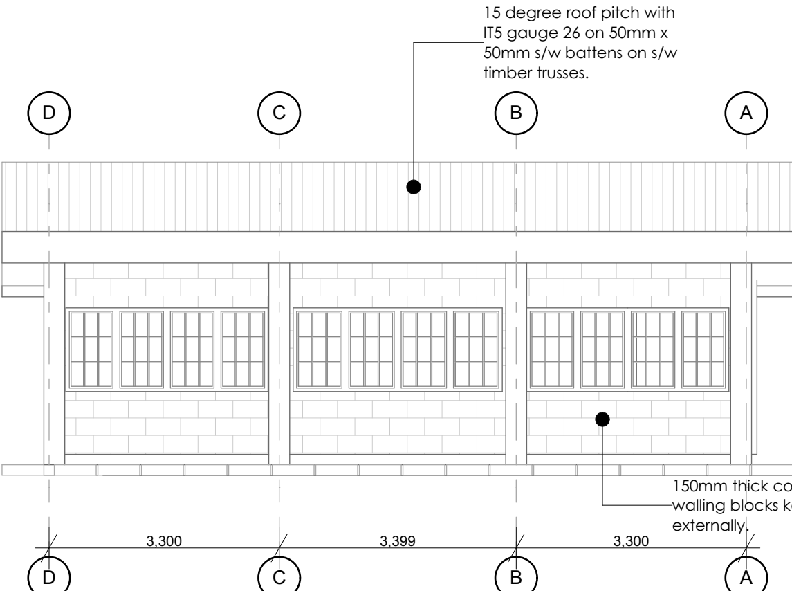
ELEVATION E-04 1:75
