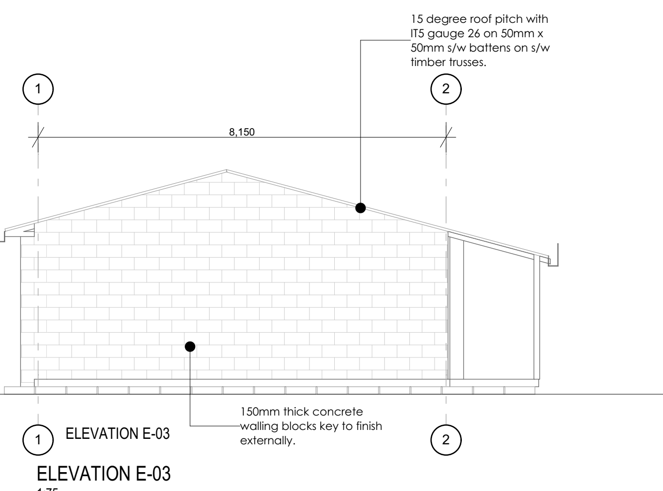
ELEVATION E-03 1:75
