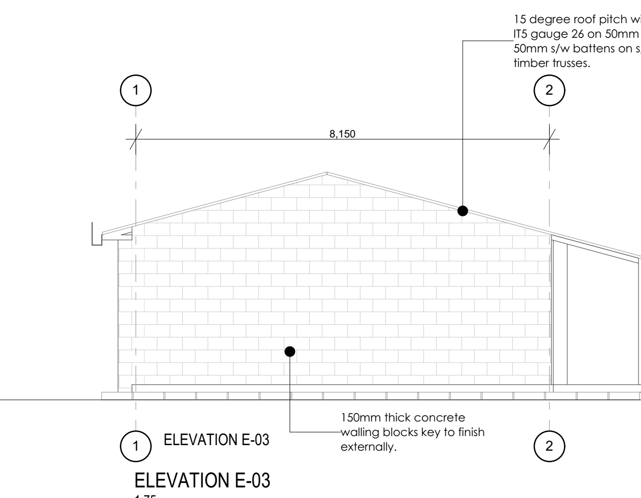
ELEVATION E-03 1:75
