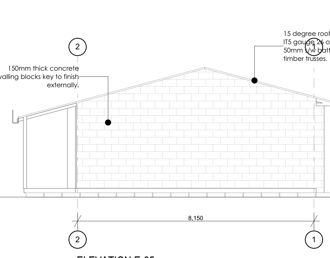
ELEVATION E-05 1:75
