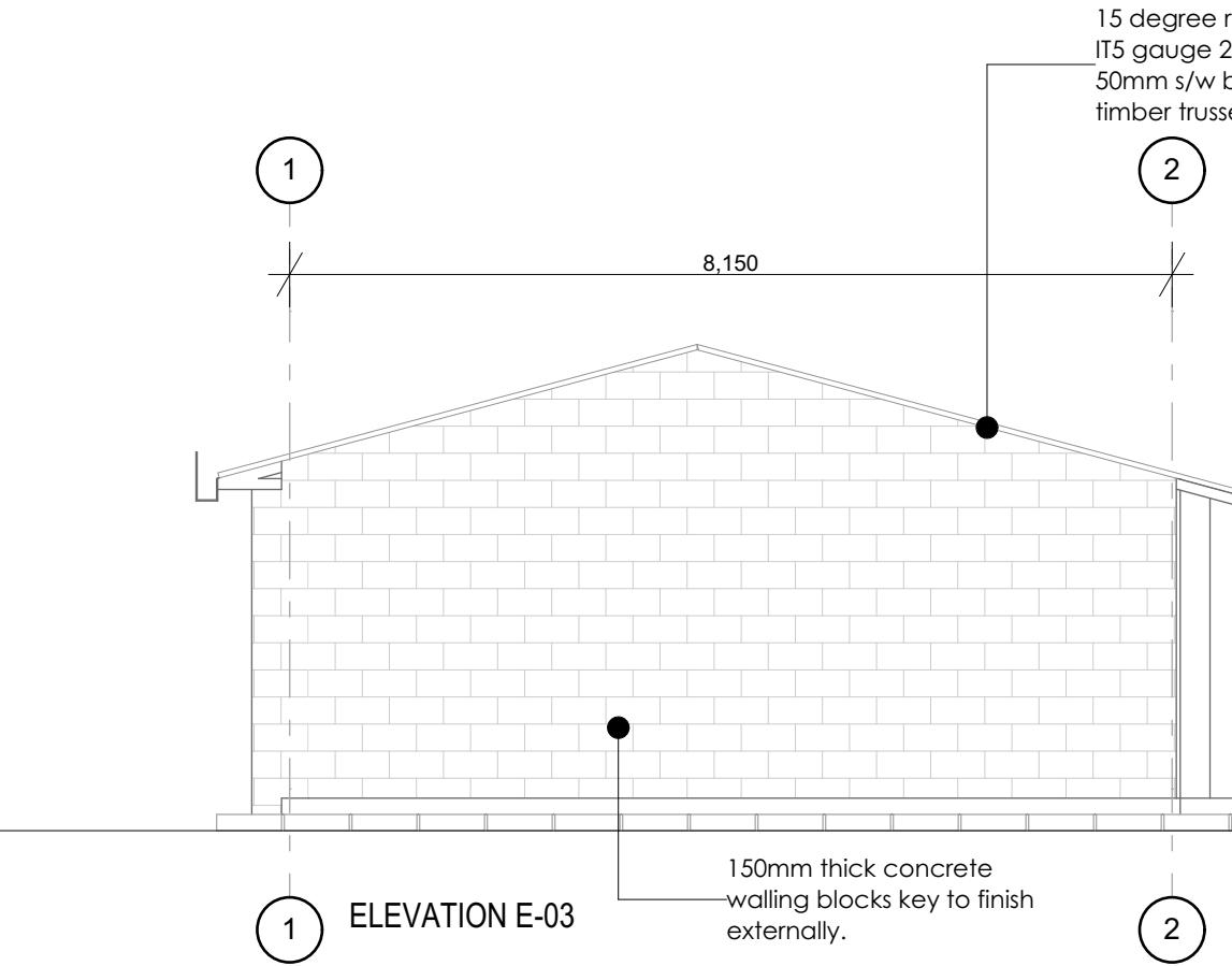
ELEVATION E-03 1:75
