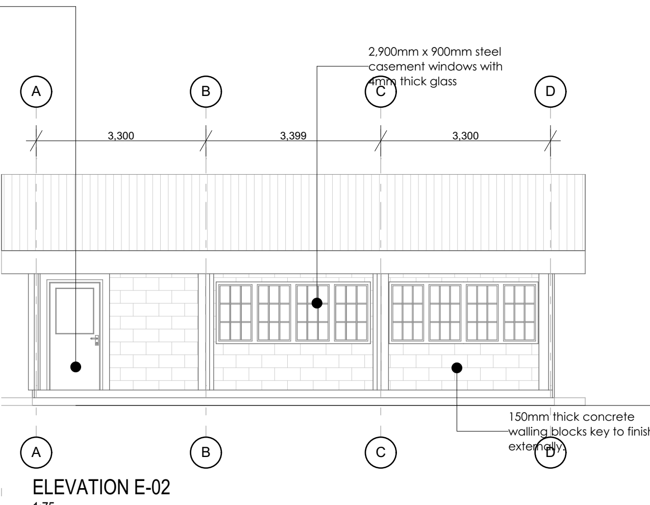
ELEVATION E-02 1:75
